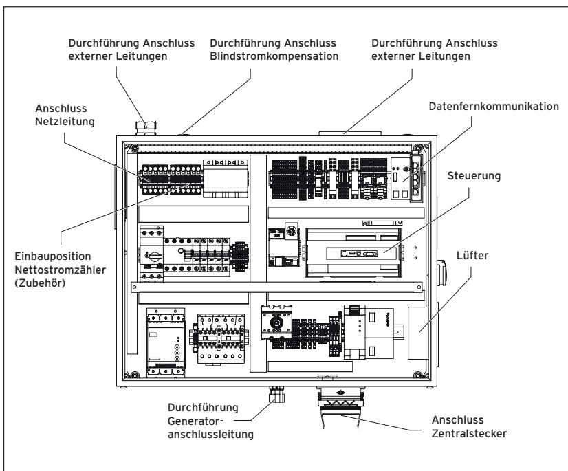
Schaltschrank (Innenansicht)
