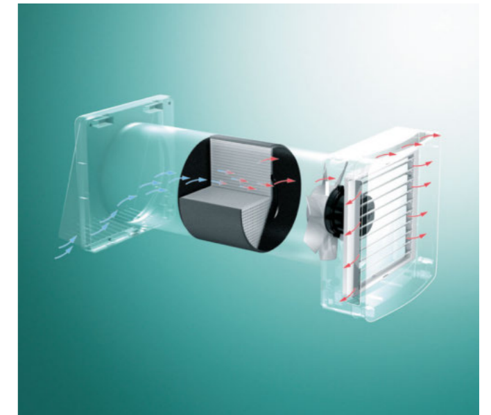
Dezentrale Lüftung recoVAIR mit Wärmerückgewinnung
